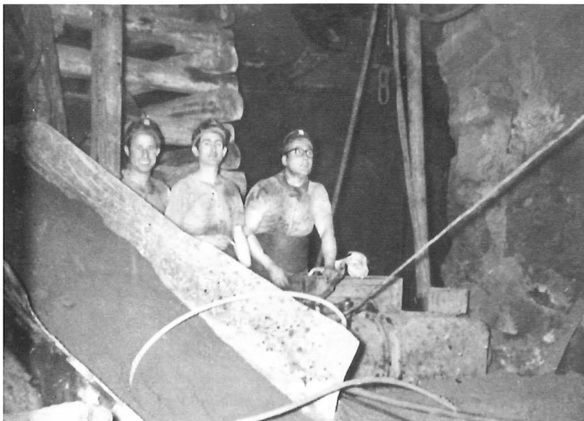
Chargeur: Boggiani Ugo avec chargeuse Estacade. Manoeuvres: Cinzio et Leone.
